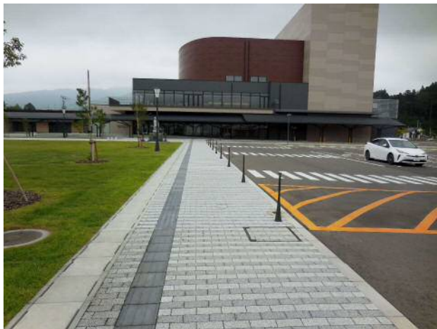
インターロッキング・陸前高田市民会館.JPG
